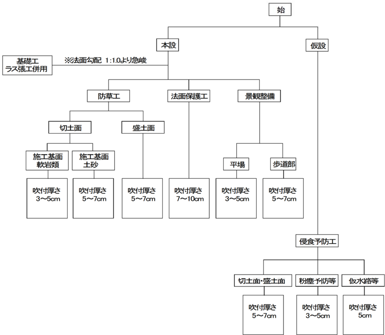
吹付厚さ 選定フロー(案)
